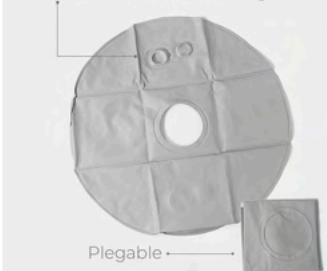
BOLSA DE CONTRAPESO Boca de relleno de arena o agua
